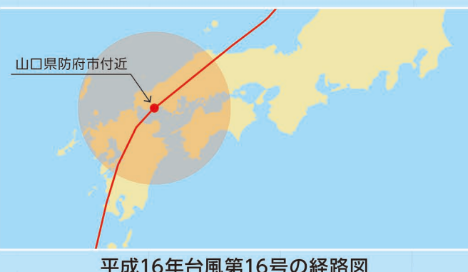
平成16年台風第16号の経路図
